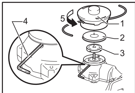
► 1. Cabeza cortadora de nailon (nylon) 2. Protector metálico 3. Arandela receptora 4. Llave hexagonal 5. Apretar
